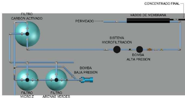
Figura 26. Propuesta 3 de tratamiento de agua captada en pozo subterráneo en área de estudio. Fuente: TECO
